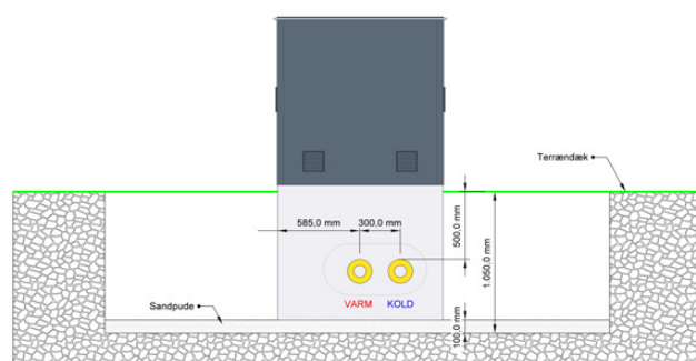
Figur 4: Driftskitse, Standard Pumpestation, returløb
