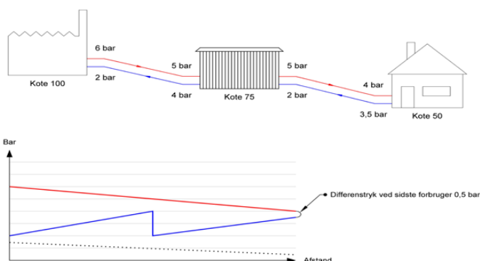
Figur 4: Driftskitse, Standard Pumpestation, returløb
