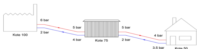
Figur 4: Driftskitse, Standard Pumpestation, returløb
