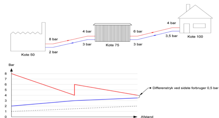
Figur 4: Driftskitse, Standard Pumpestation, returløb
