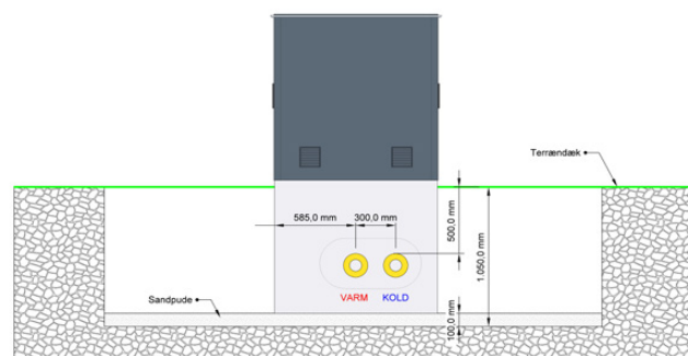
Figur 4: Driftskitse, Standard Pumpestation, returløb
